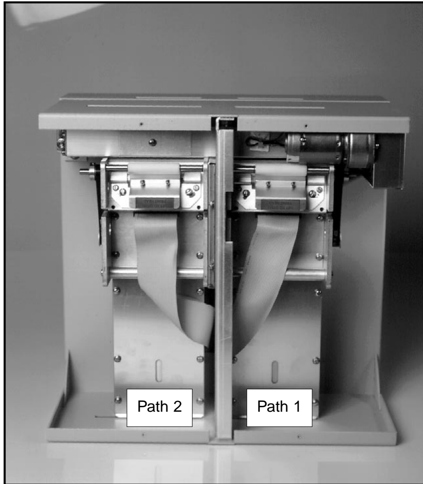
Figure 3 - Dual Mini - Top view
