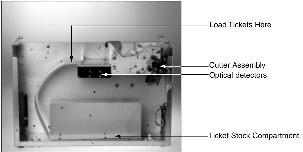
Figure 3a - Mini Plus side view
